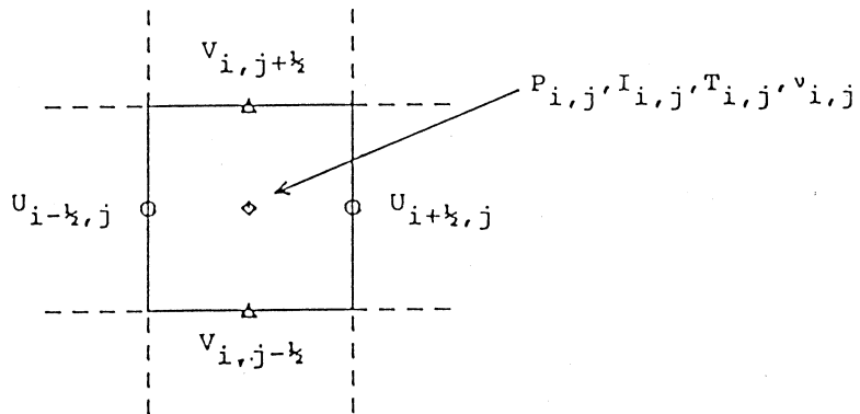
図4 格子における物理変数の配置
